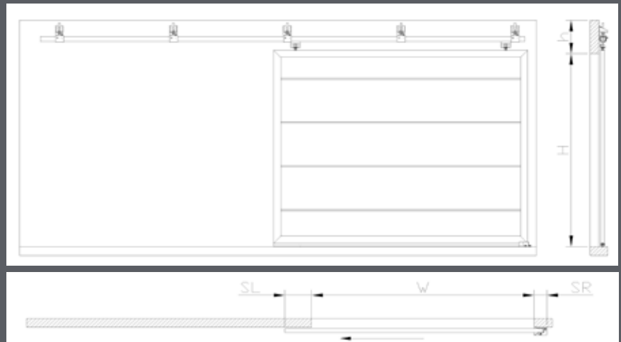
Side lock or floor lock options/ Seitenverriegelung - optional Bodenverriegelung
